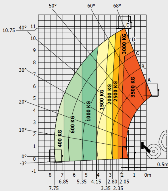
Maschine auf Rädern mit Gabelzinken
