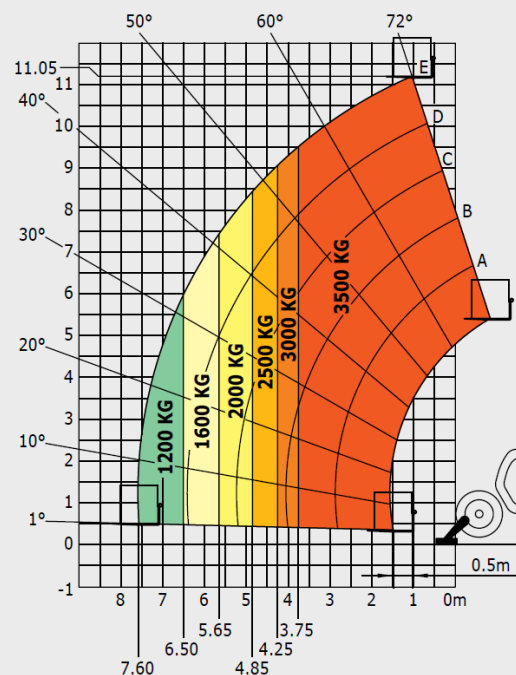
Maschine auf Stützen mit Gabelzinken
